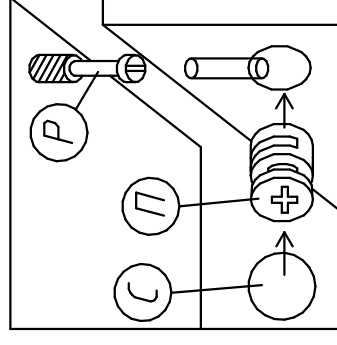
Крепление стяжки эксцентриковой (комплект №45)
